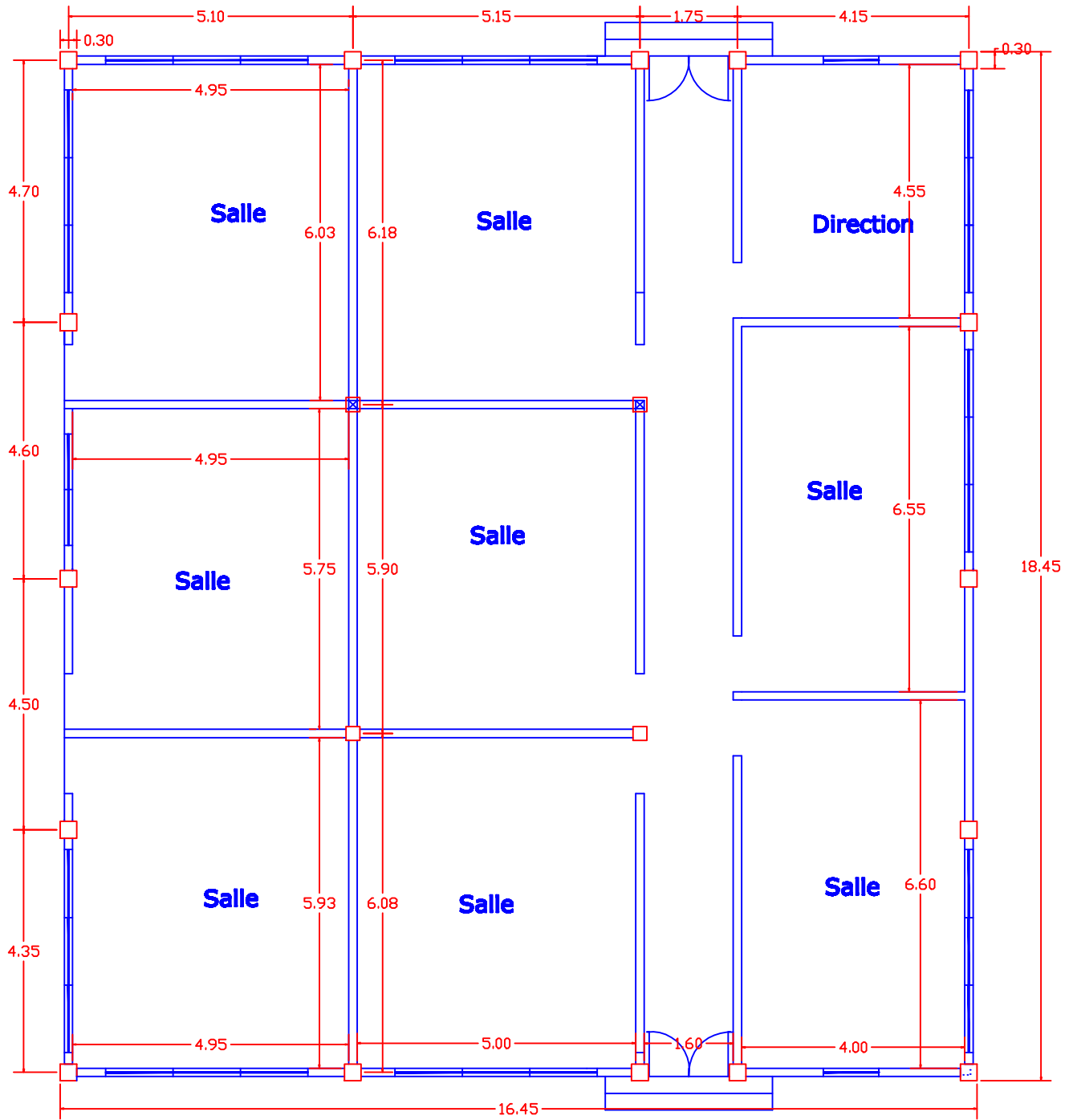
VUE EN PLAN BATIMENT
